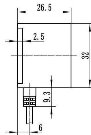
图 2. HPS-166C-L 侧视图
